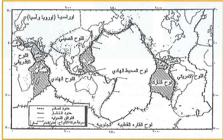
شكل (١): الصفائح الصخرية المكونة للقشرة الأرضية
