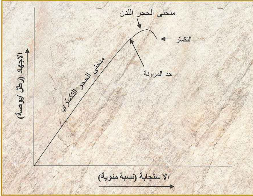
(شكل ١) العلاقة البيانية بين الاجهاد والاستجابة
